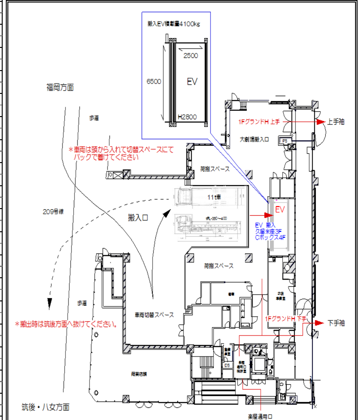
搬入口平面図
